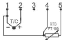
2x termočlánek
