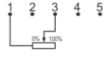
Potenciometr, 3-vodič
